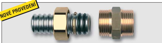
Art. Y5442x přechodka na vnější závit pro trubku TFG (plyn)
